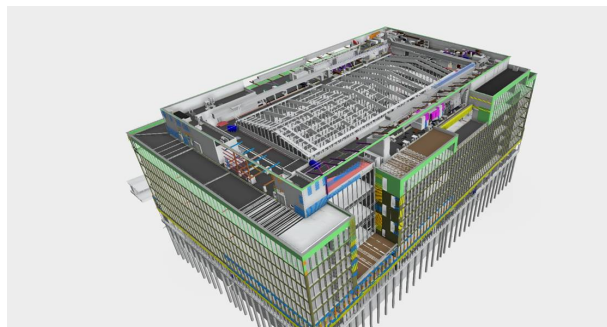
La maquette BIM de Pulse : 28.000 m 2 de bureaux à Saint-Denis (Janvier 2019)
